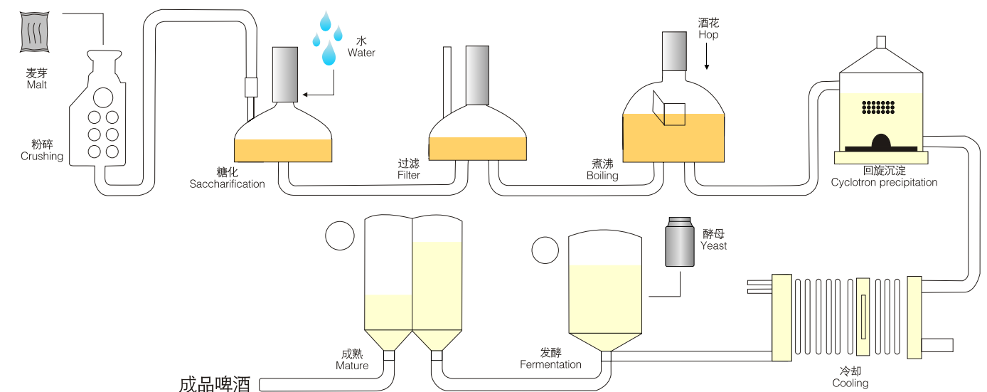
鲜啤酒吧工艺流程图
